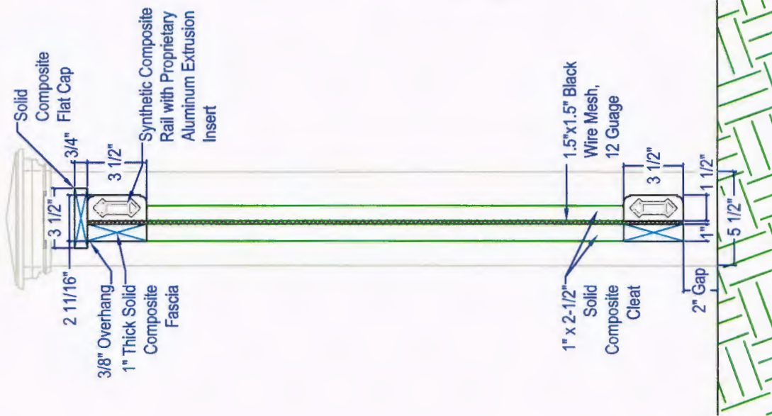
2 Fence Section Scale: 1-1/2" = 1'-0"
